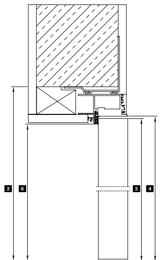
Navpični prerez s površinsko izravnanim vratnim krilom
