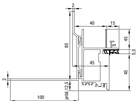
Dimenzioniranje podboja Zeroline
