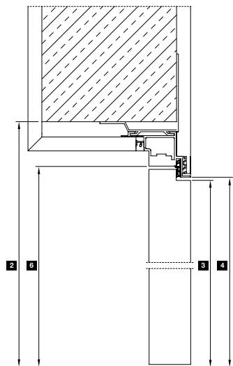
Navpični prerez z vratnim krilom, ki se odpira vzvratno
