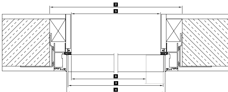
Vodoravni prerez s površinsko izravnanim vratnim krilom
